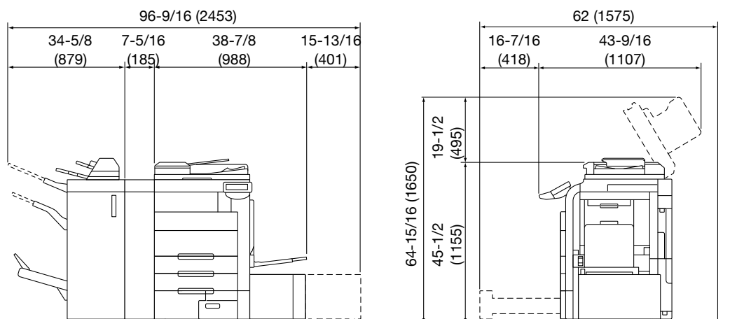
ineo+ 552/652 + FS-526 + SD-508 + ZU-606 + PI-505 + LU-301 Единица измерения: дюйм (мм)
