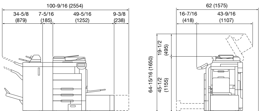
ineo+ 552/652 + FS-526 + SD-508 + ZU-606 + PI-505 + LU-204 Единица измерения: дюйм (мм)
